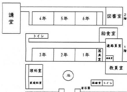
昭和42年度 飯谷小学校校舎平面図
